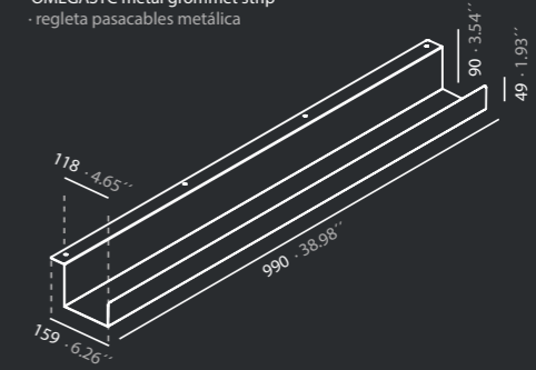
OMEGASTC metal grommet strip · regleta pasacables metálica
